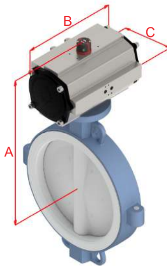
Actuador neumático doble efecto Double acting actuator
